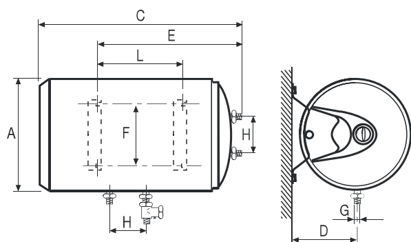
Fig. 3 .- Modelos TNC plus 30 S,TNC plus 50,TNC plus 50 S, TNC plus 80,TNC-80 S,TNC plus 100, TNC plus 150
